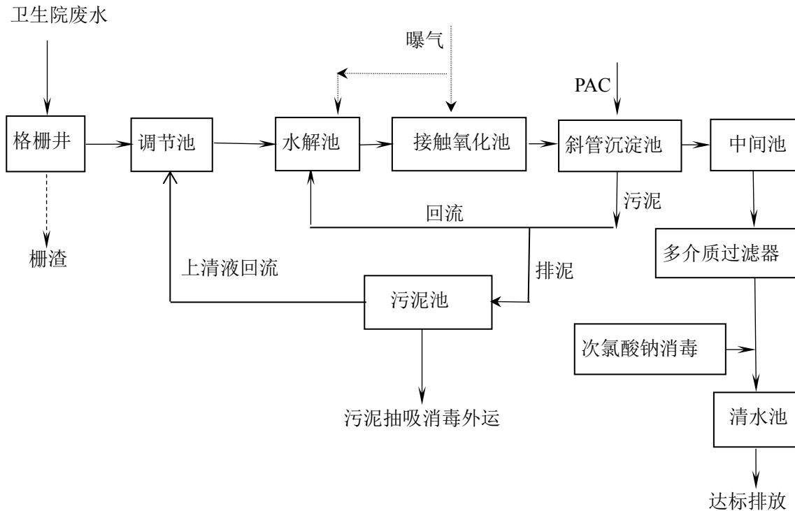
图 4-1 水磨镇卫生院污水处理站工艺流程图
